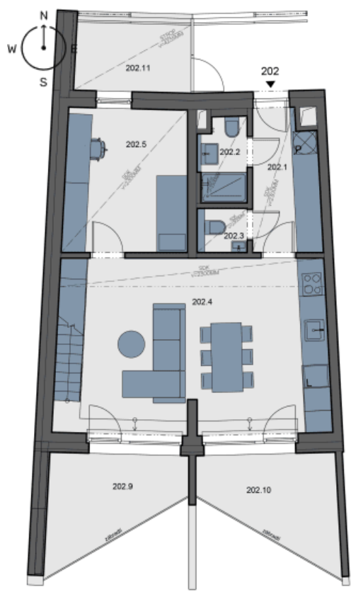
Půdorys podlaží
