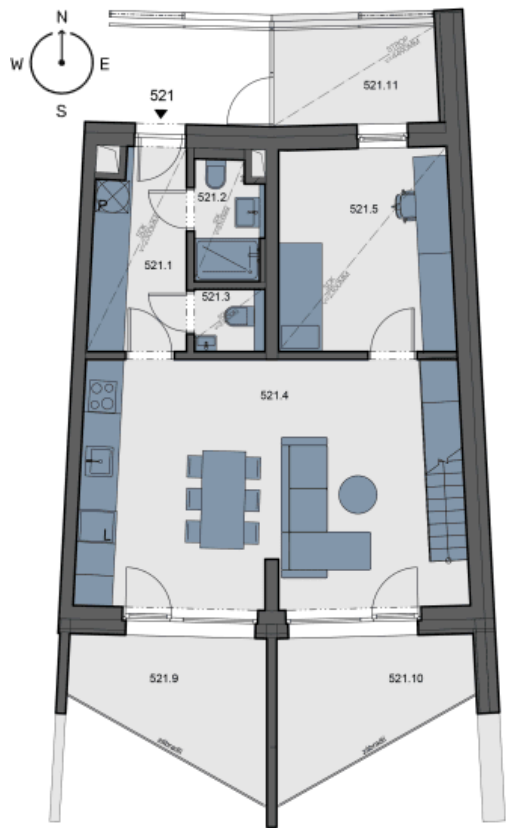
Půdorys podlaží
