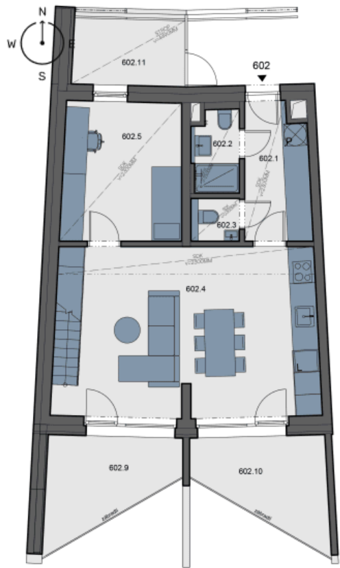
Půdorys podlaží
