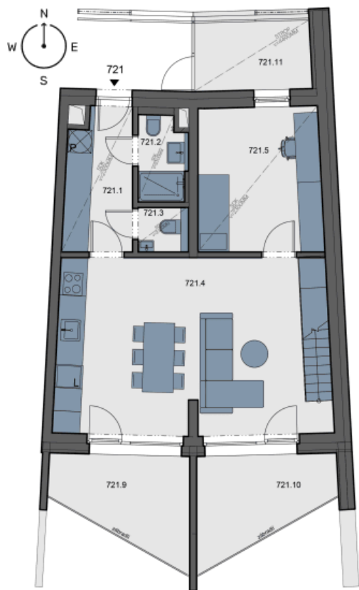
Půdorys podlaží
